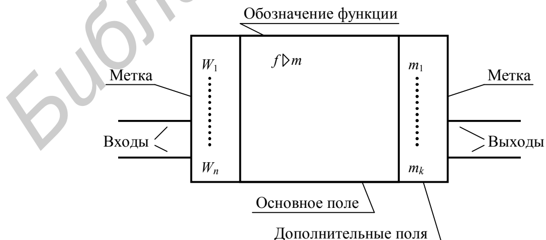
Рисунок 3.16 – Условное графическое обозначение элементов аналоговой техники (к пункту 3.5.2)
