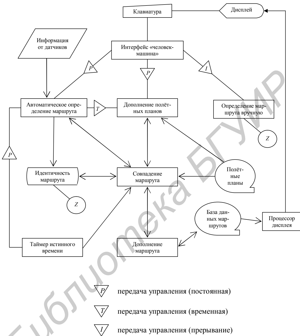
Рисунок 3.31 – Схема взаимодействия программ
