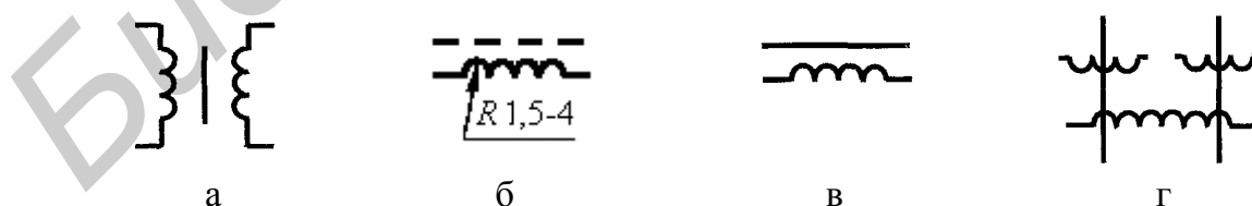
Рисунок 3.5 – Условные графические обозначения трансформатора, катушки индуктивности, дросселя и магнитного усилителя (к пункту 3.3.1)
